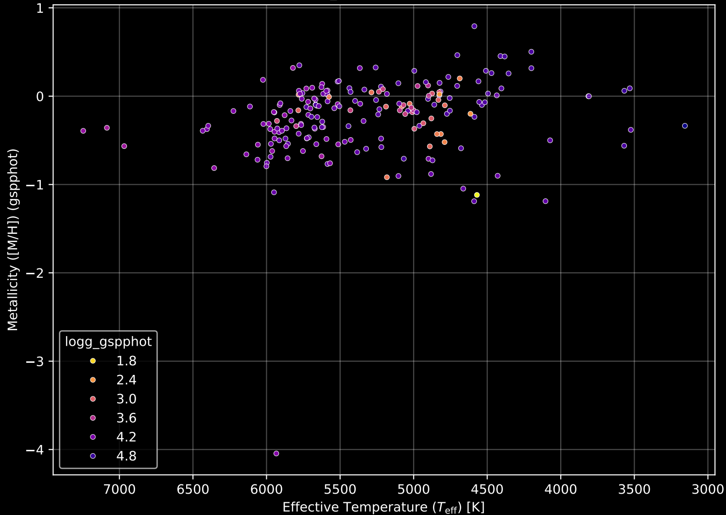
APOGEE DR17 Field: [114+62_MGA] Stellar Population Parameters (n= 200)
